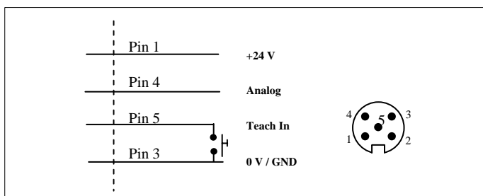
Wiring/Anschlüsse/Raccordement électrique
